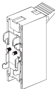
FIJACION CON BRIDA METÁLICA "BO" PARA CARRIL
